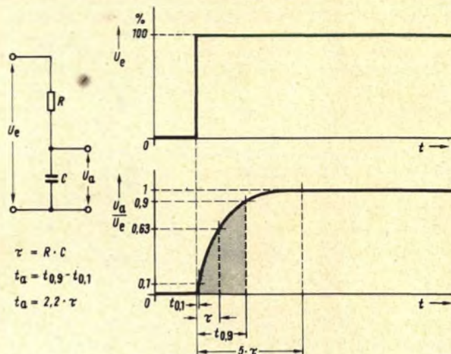
Bild 5.13. RC-Tiefpaß, Anstiegszeit und Zeitkonstante
