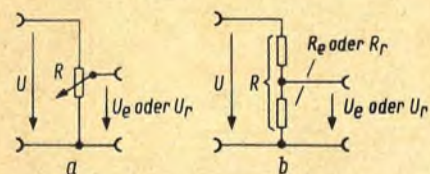
Bild 1. Potentiometer (a) und Ersatzschaltung (b)
