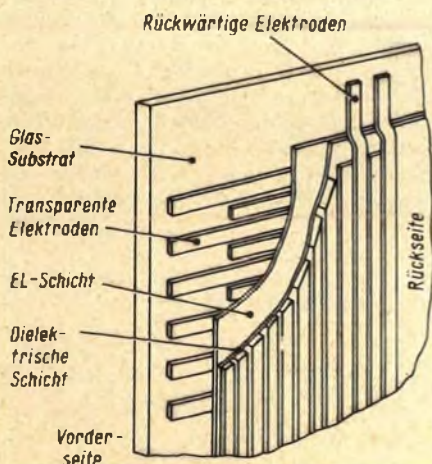
◀ Bild 1. Der flache „Sandwich“ des EL-Bildschirms von Mitsubishi mit Elektrodenlamellen und Zwischenlagen
