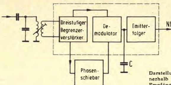
◀ Bild 43. Prinzipschaltung des Z_f -Verstärkers mit Koinzidenzdemodulator. Alle Stufen innerhalb der gestrichelten Umrandung befinden sich innerhalb des integrierten Siliziumbausteines
