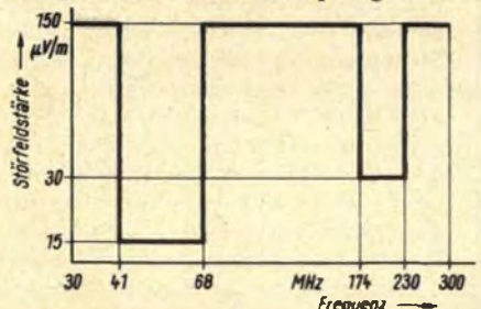
Zulässige Störfeldstärke von UKW-Empfängern im Bereich 30...300 MHz, gemessen in 30 m Entfernung
