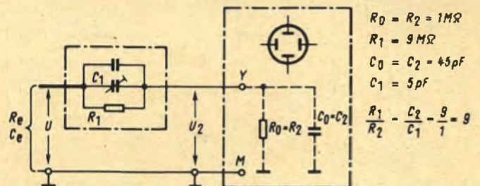
Bild 5.9. Oszilloskop mit Tastkopf und frequenzkompensiertem Spannungsteiler
