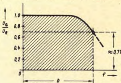
Bild 5.12. RC-Tiefpaß. Grenzfrequenz und Bandbreite
