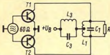
Bild 2. Wirkungsgradverbesserung bei einer Gegentakt-Endstufe
