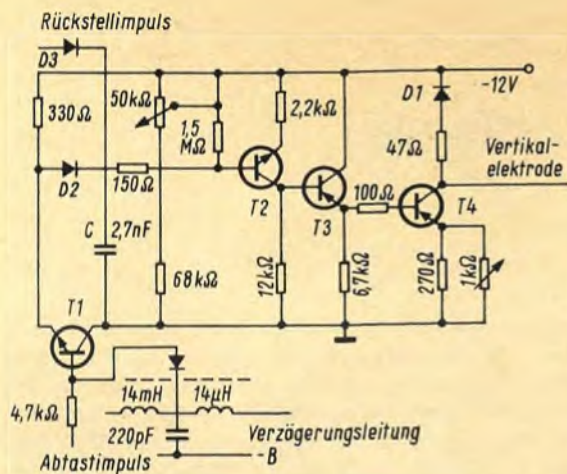
Bild 3. Die Schaltung zur Helligkeitssteuerung beim Matushita-Schirm. An jedem der 230 Abgriffe der Verzögerungsleitung befindet sich diese Steuereinheit
